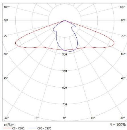
Krivka svietivosti v polárnych súradniciach
